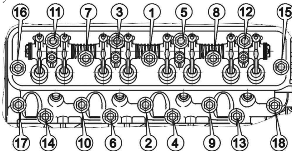
Рис.14. Порядок подтяжки гаек крепления головок цилиндров
