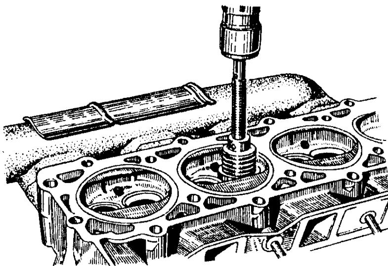
Рис.62. Обработка седел клапанов
