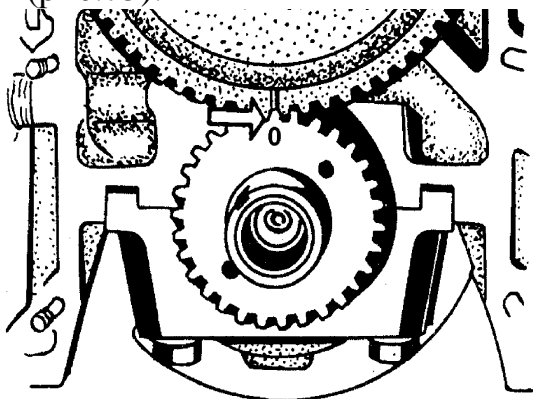
Рис.75. Установка шестерен распределения:
