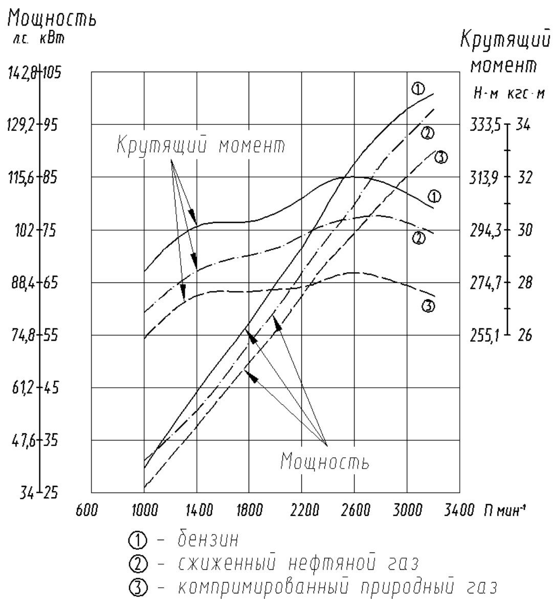
Рис.8. Внешняя скоростная характеристика двигателя брутто
