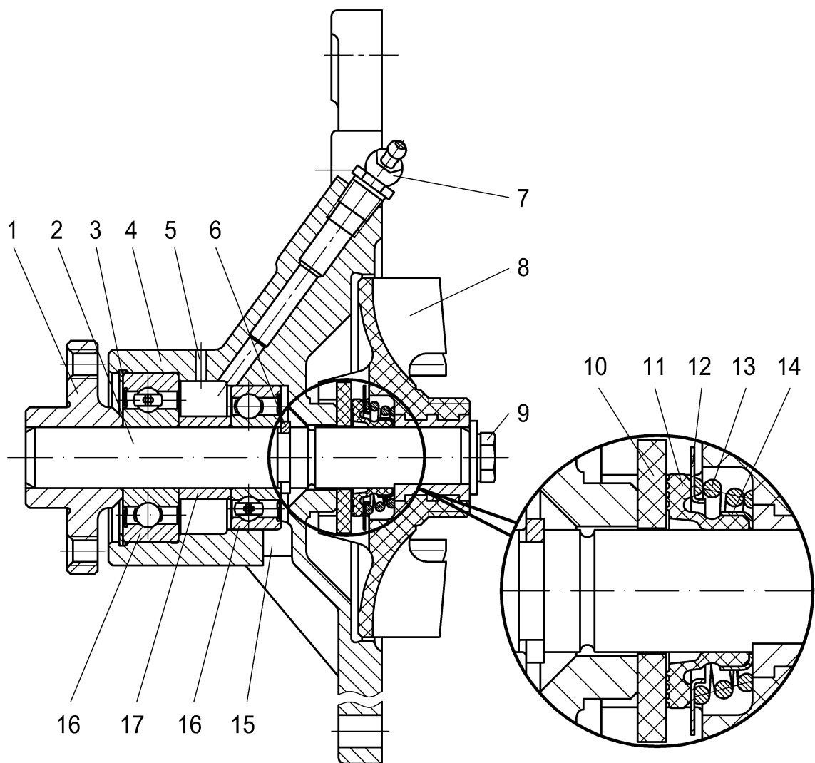
Рис.26. Водяной насос с уплотнением старого образца:
