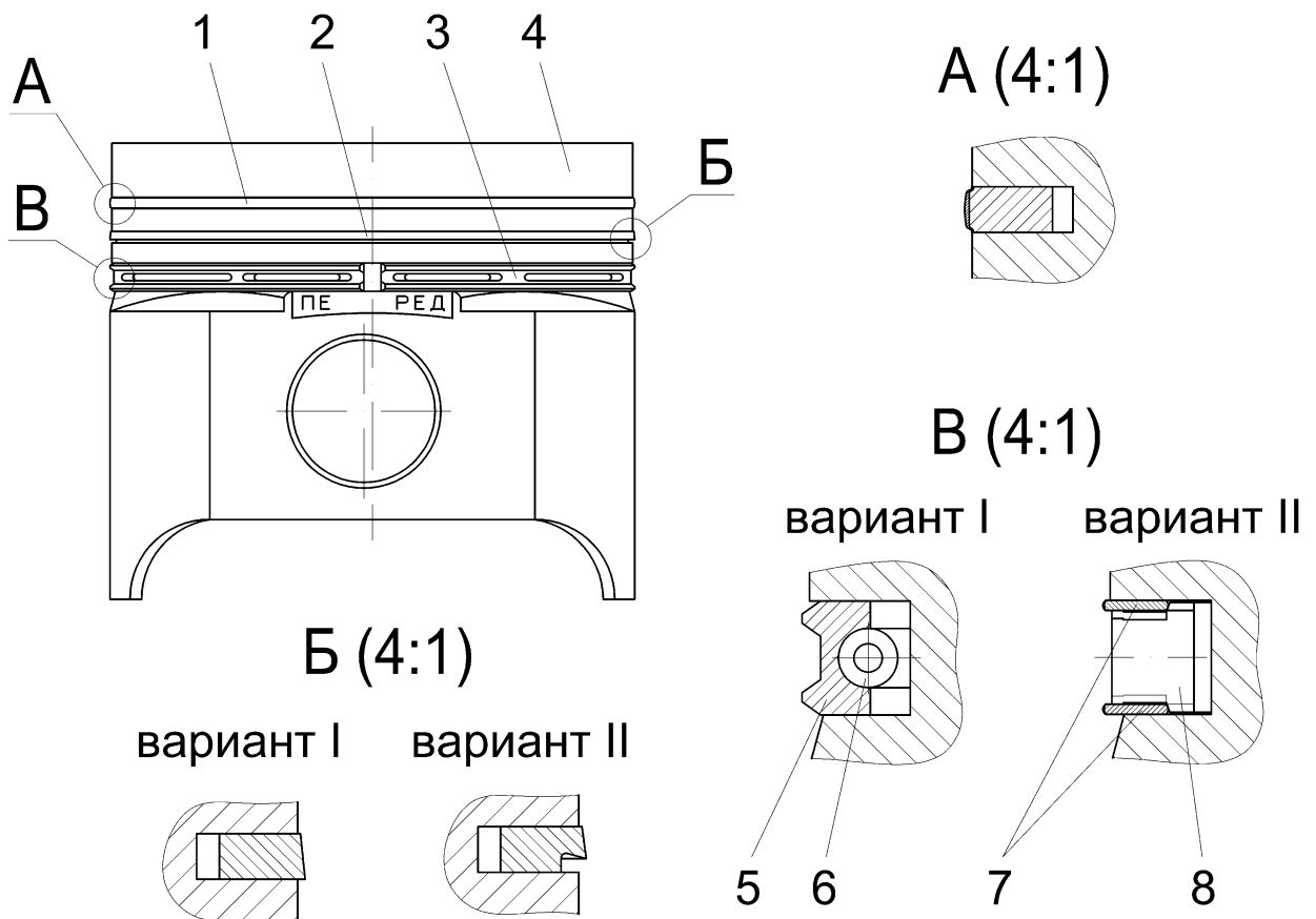
Рис.11. Поршневые кольца:
